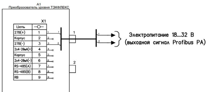
Рисунок Г.5 - Схема электрическая подключения преобразователя исполнения PA
