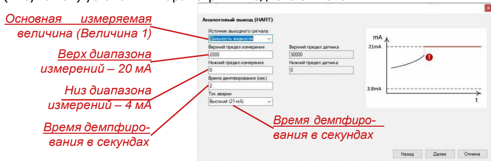
Рисунок 52. Параметры выходного сигнала 1
