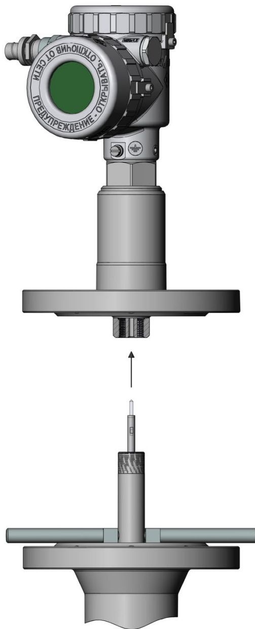
Рисунок М2.3 - Отсоединение Тэкфлекса от процесса
