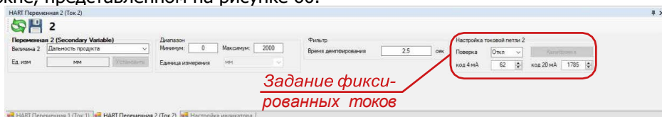
Рисунок 60. Формирование фиксированных значений тока по выходу 2
