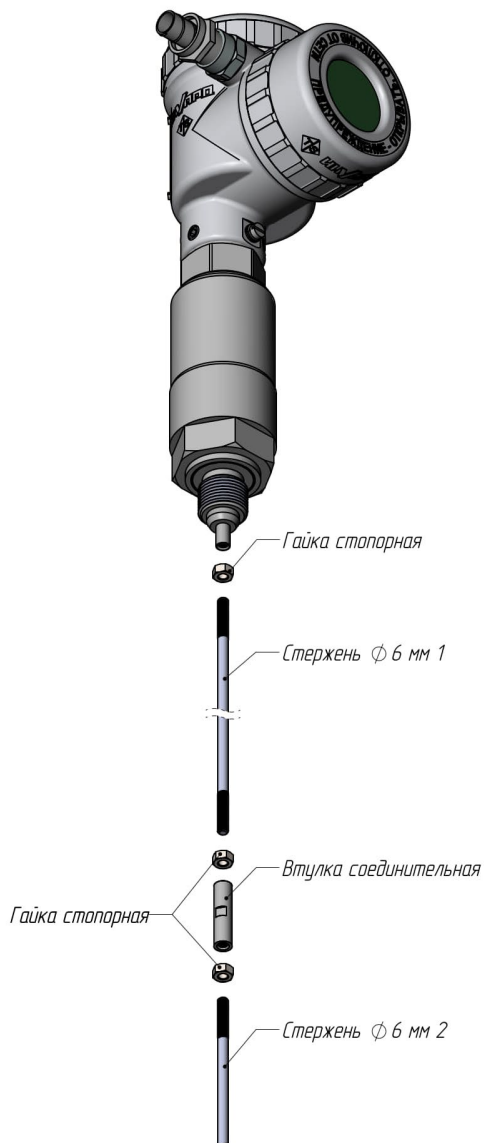
Рисунок Е16 – Монтаж составного жесткого зонда из стержня Ø6 мм
