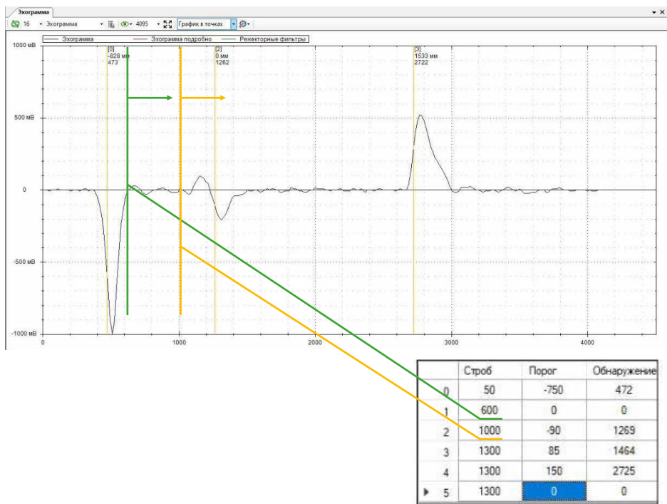
Рисунок 21. Задание стробов обнаружения перехода 1 и 2
