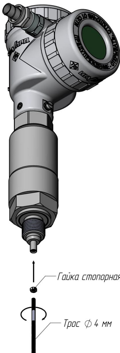
Рисунок Е14 – Монтаж одиночного гибкого зонда
